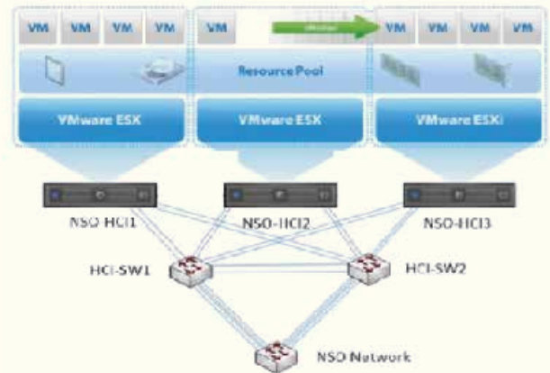
รูปแสดงสถาปัตยกรรมระบบ Private Cloud NSO
