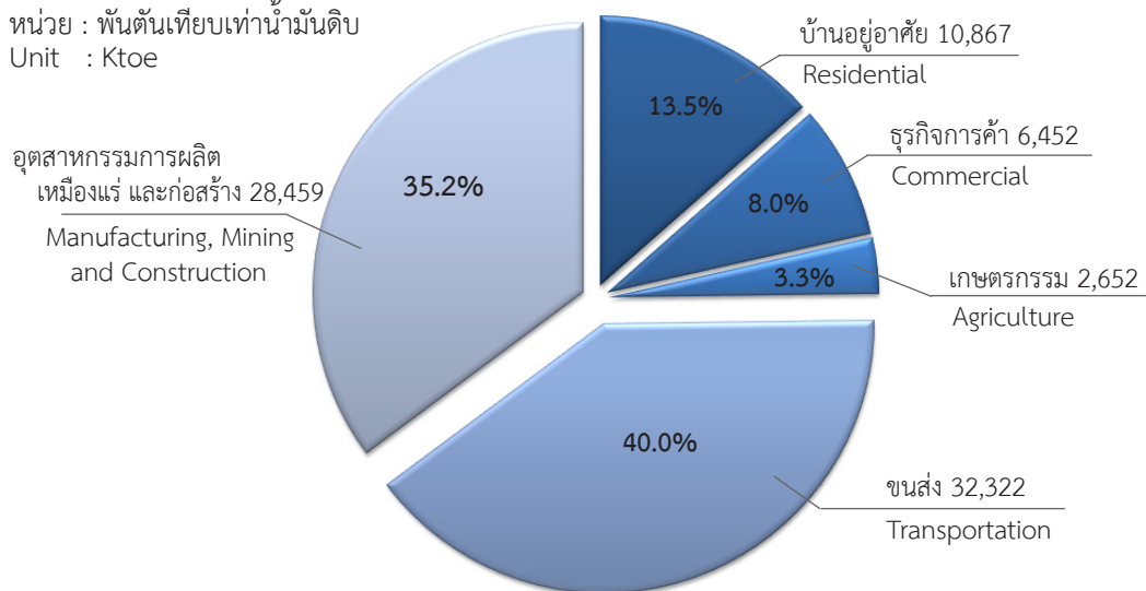
แผนภูมิ 4.2 การใช้พลังงานขั้นสุดท้าย จำแนกตามสาขาเศรษฐกิจ พ.ศ. 2560 Chart 4.2 Final Energy Consumption by Economic Sectors: 2017
